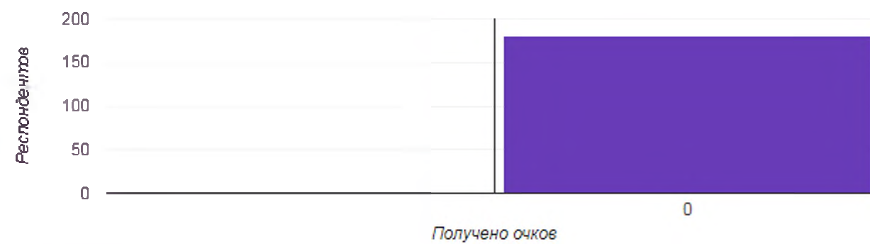
Распределение баллов
